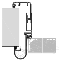
EUROFI Umfassungszarge
