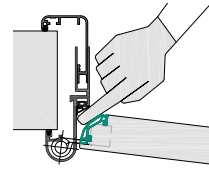
Nachgiebige Knautschzonen
