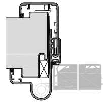
RENOFI Renovierungszarge
