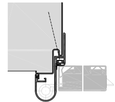
EFI Renovierungs-Eckzarge über bestehender Stahlzarge
